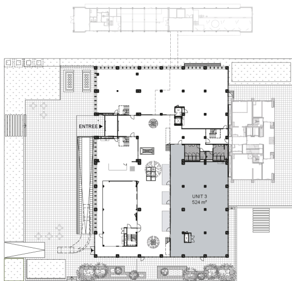
BEGANE GROND
